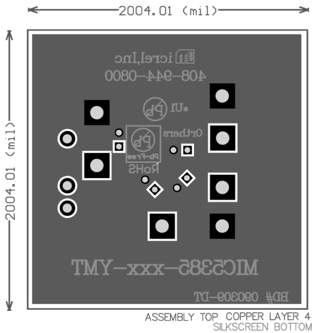
Bottom Layer
