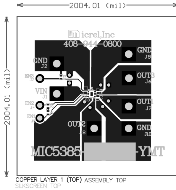
Top Layer
