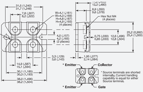
ISOTOP® or SOT-227
