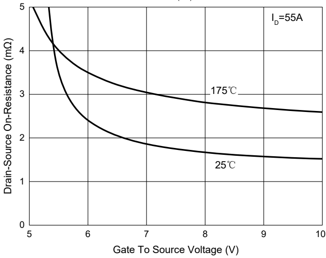
Fig. 3 - R_{DS(ON)} - V_{GS}
