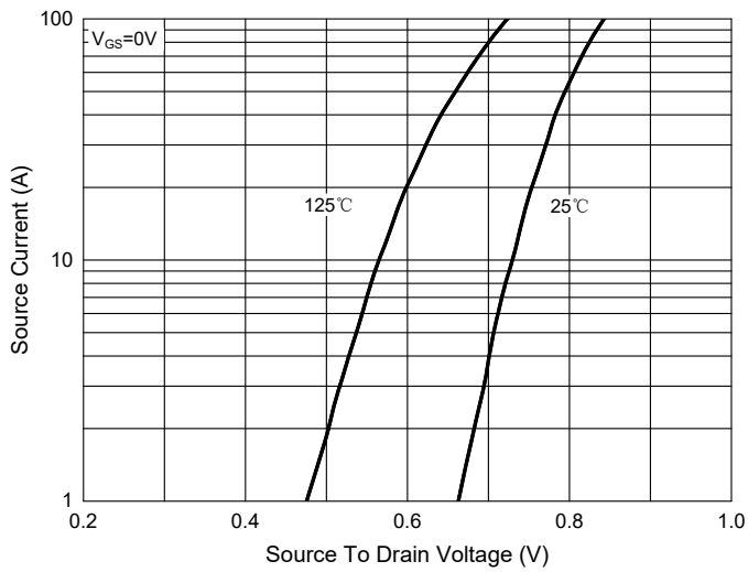
Fig.9 - I_s - V_{SD}
