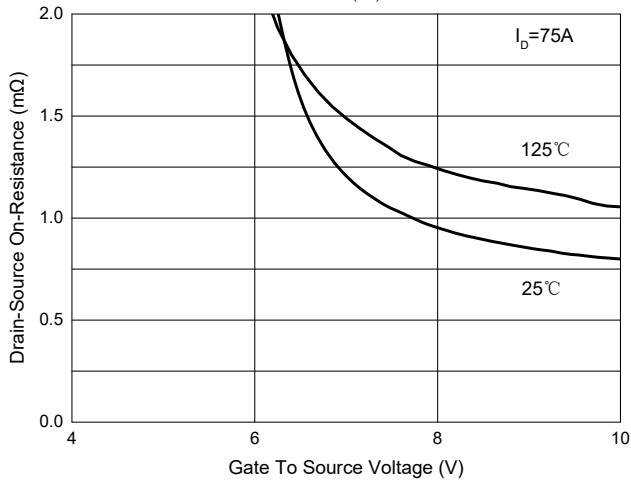
Fig. 3 - R_{DS(ON)} - V_{GS}
