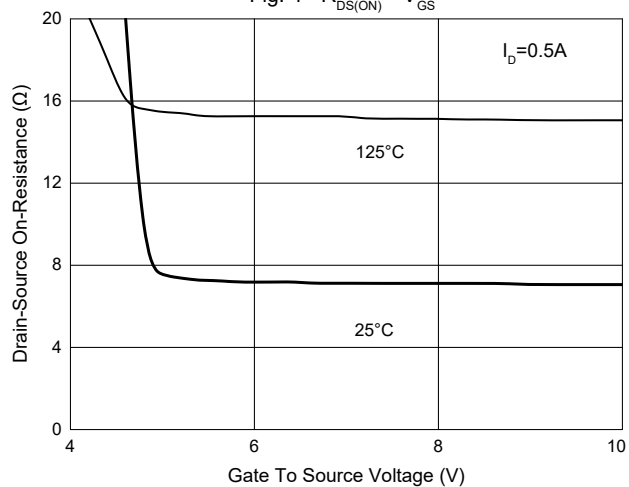
Fig. 4 - R_{DS(ON)} - V_{GS}
