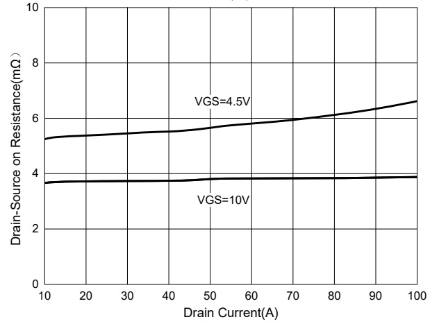
Fig. 4 - R_{DS(ON)} - I_D
