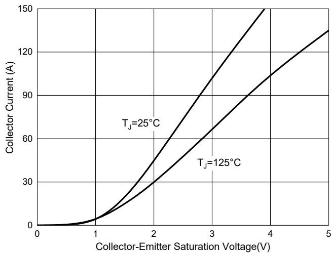
Fig. 5 - V_{CE(sat)} - I_C
