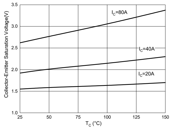
Fig. 6 - V_{CE(sat)} - T_C
