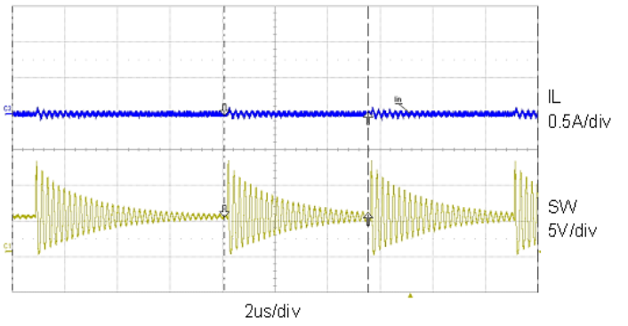
PFM switching
