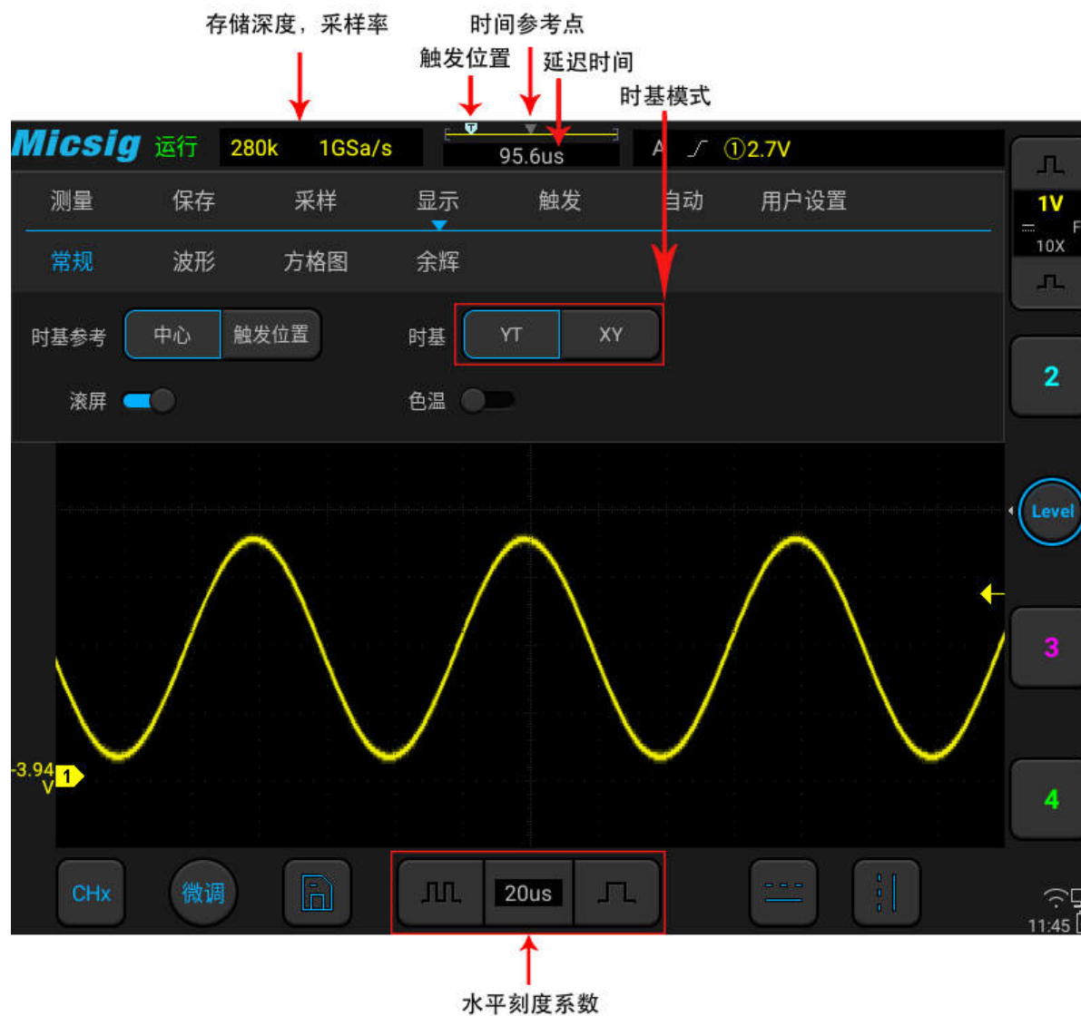
图4-1 水平系统
