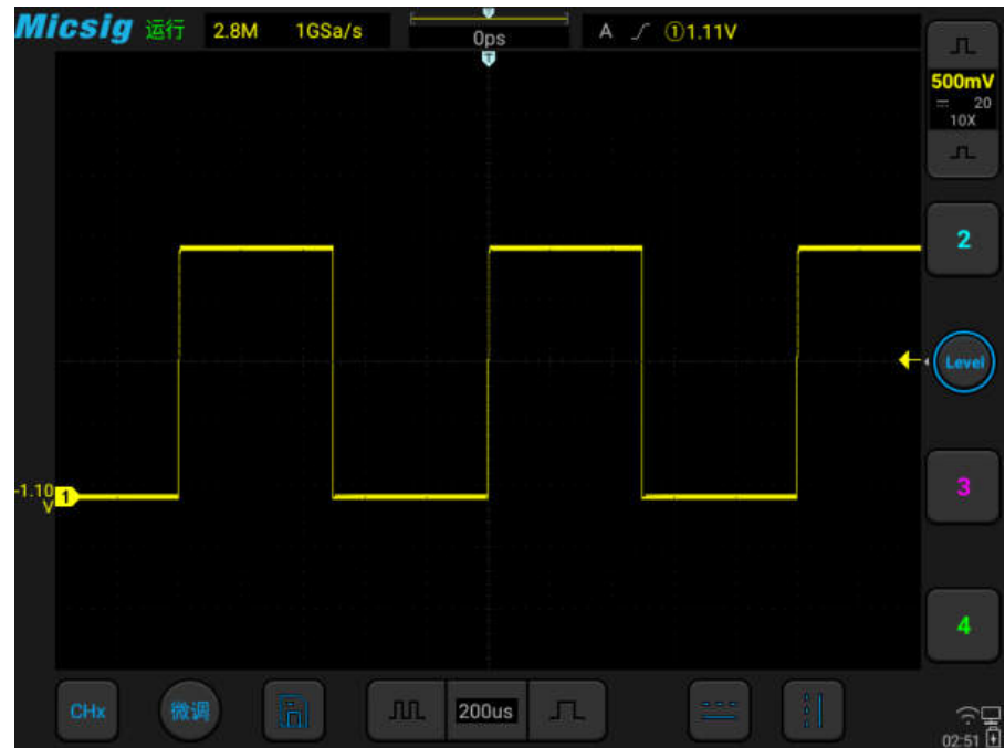
图5-11 20M带宽
