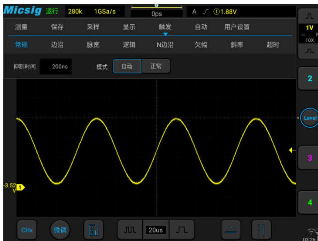
图6-5 示波器触发模式设置
