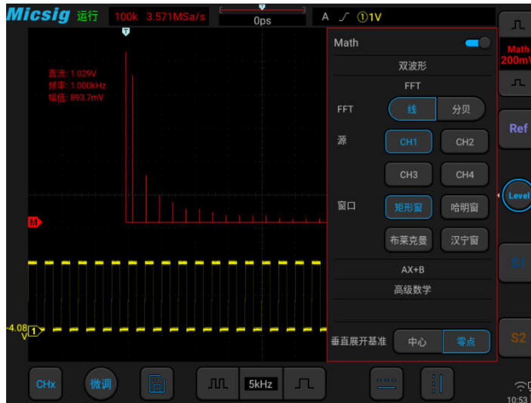
图9-3 FFT 窗口
