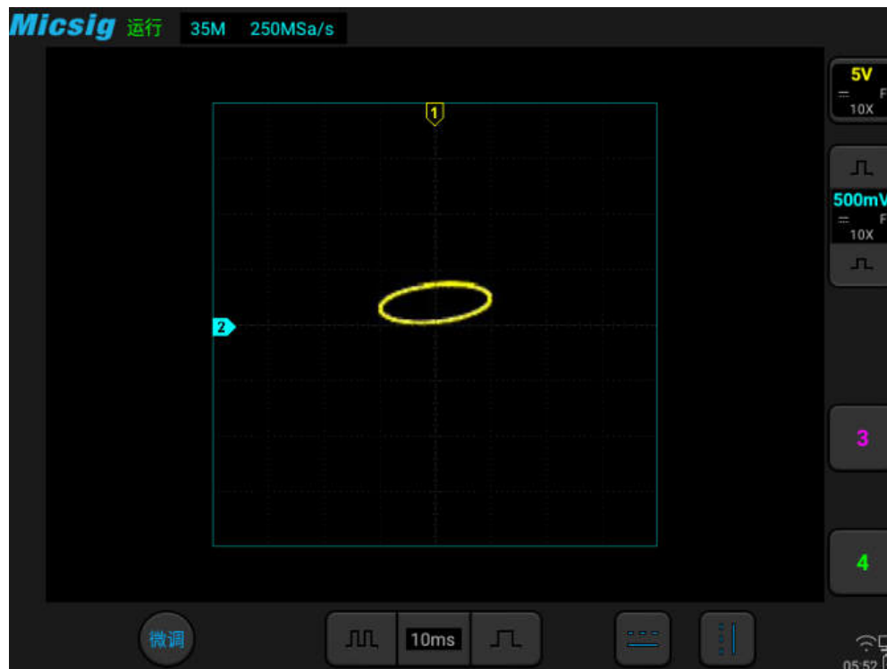
图4-8 XY 模式
