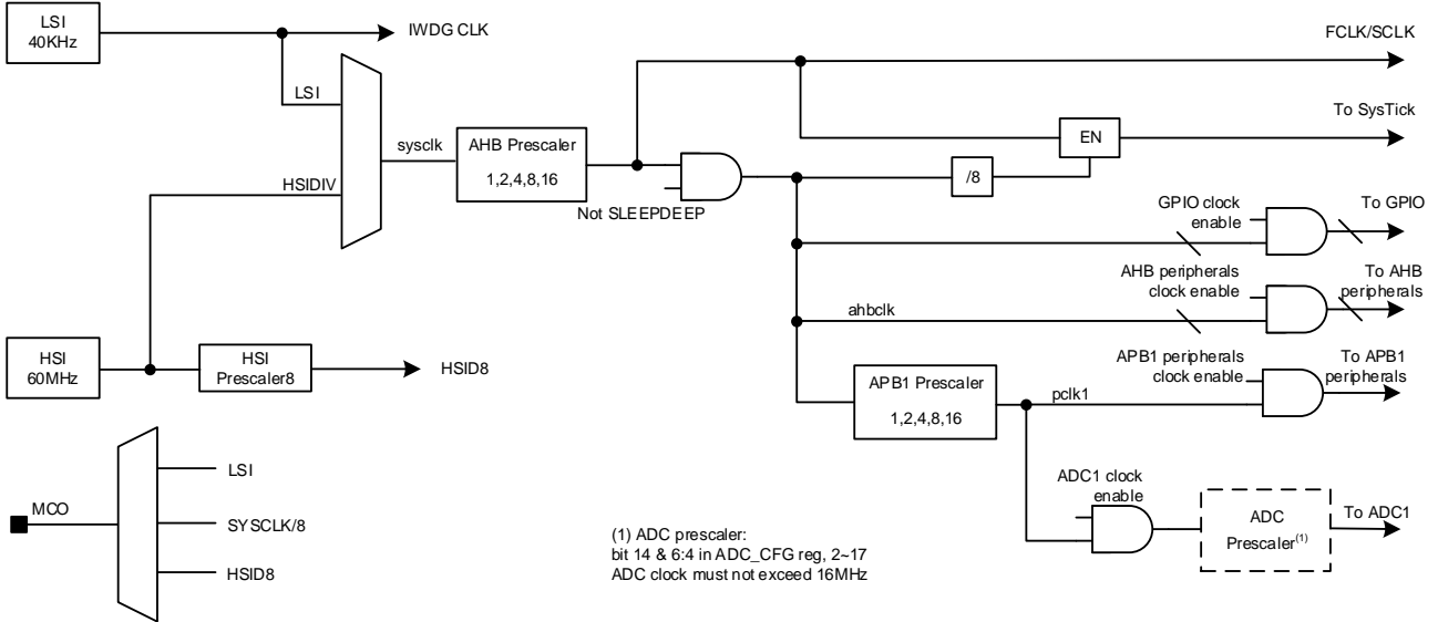
图 4 时钟树
