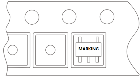
SOT23-5 示意图
