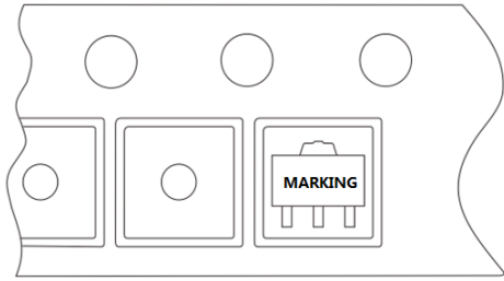
SOT89-3 示意图
