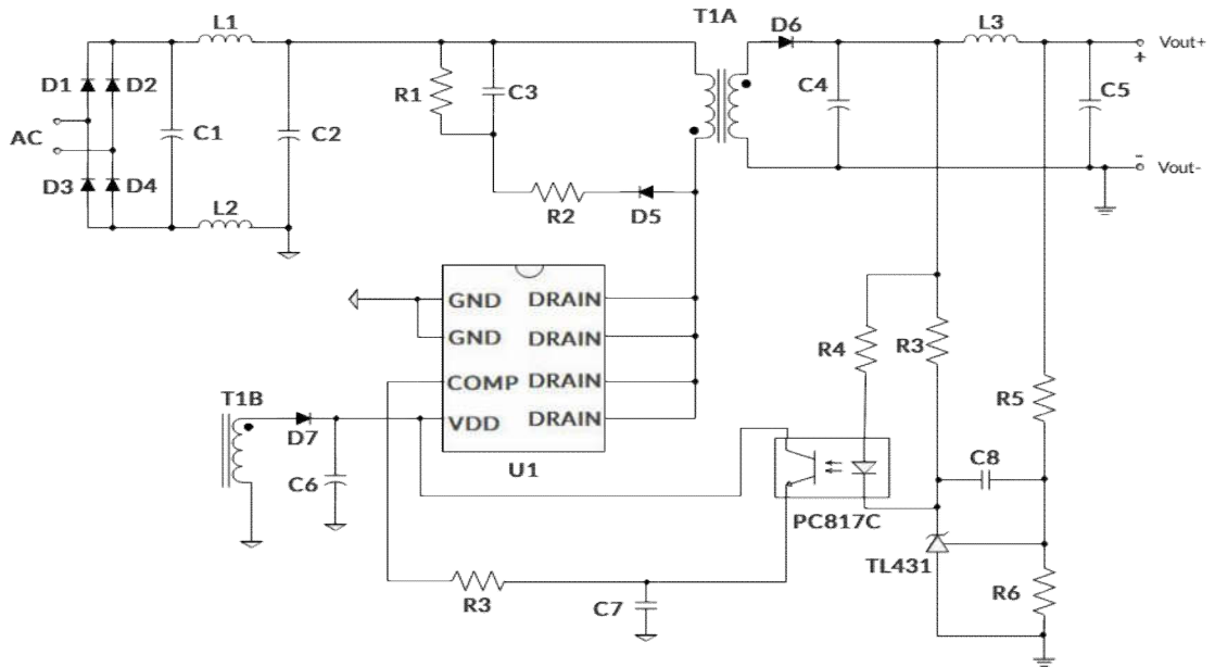
图 2 典型应用图
