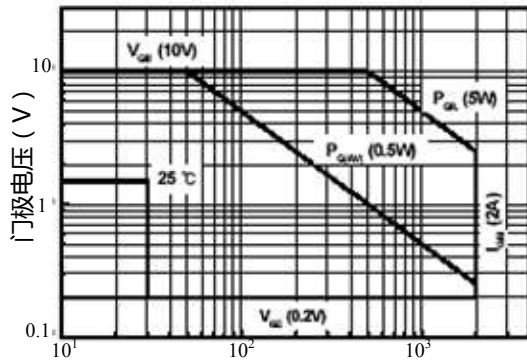
图一、门极特性
