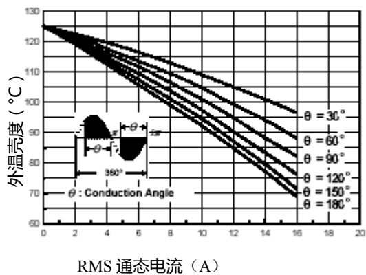
图五、通态电流---外壳温度
