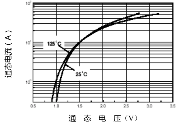
图二、通态电压
