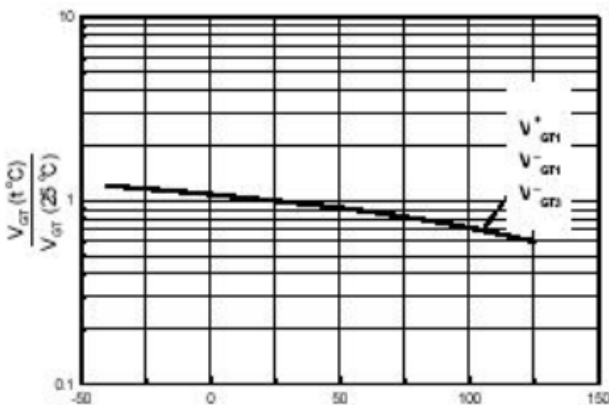
结温 (°C)
