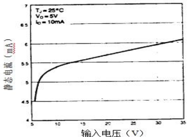
静态电流
