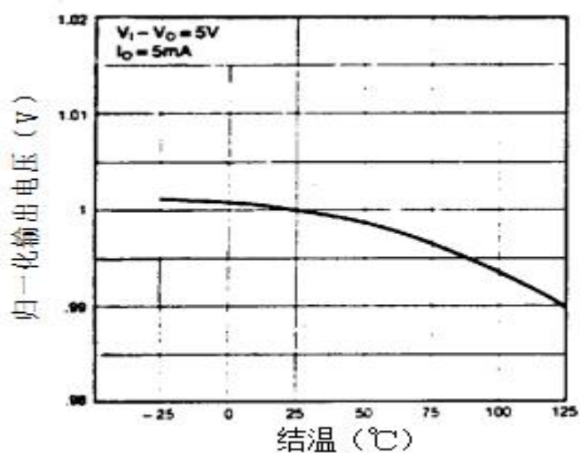
输出电压
