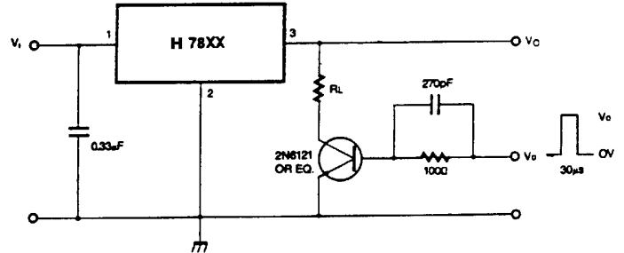
图 2、负载调整率测试
