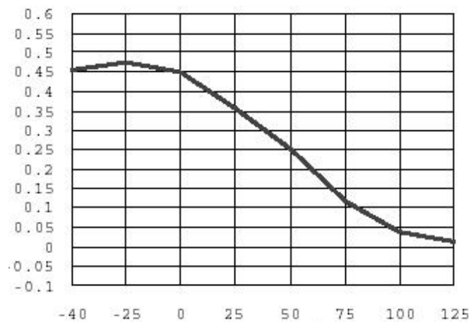
图5 短路电流
