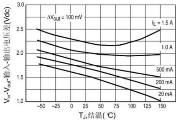
图 5. 电压压降 Figure 5. Dropout Voltage
