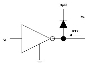
图10、 I_{CEX} 测试电路
