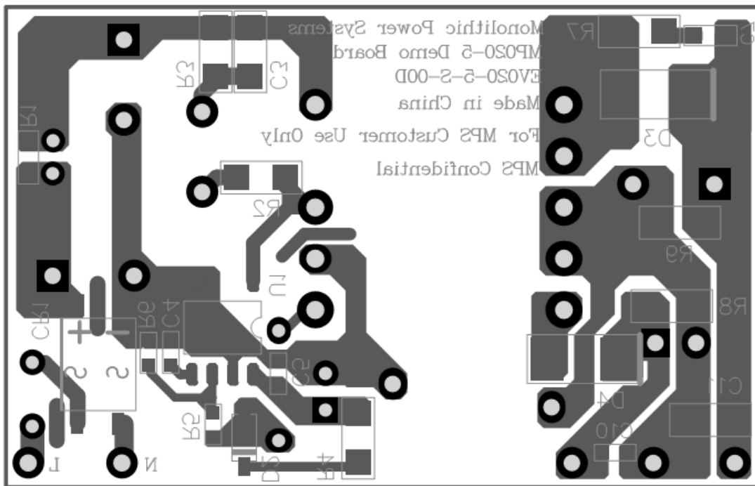
Figure 3—Bottom Layer
