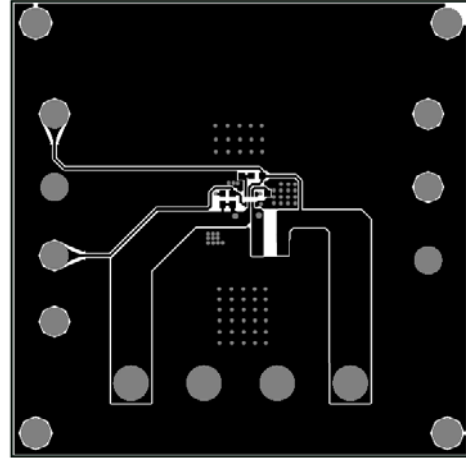
Figure 4—Top Layer
