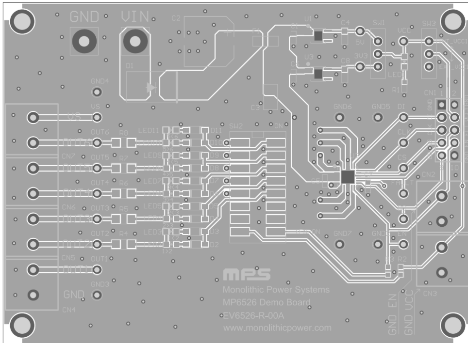
Figure 1—Top Layer
