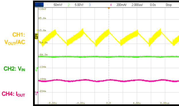
V_{OUT} Ripple
