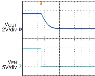
EN Shutdown Waveform
