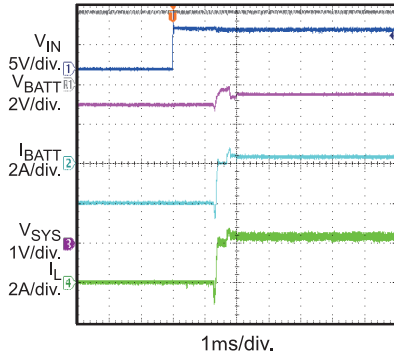
Plug in Adapter V_{BATT} = 3.7V , I_{SYS} = 2A
