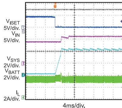
Charge On V_{IN} = 9V , No Battery, I_{SYS} = 3A
