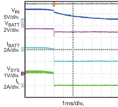
Remove Adapter V_{BATT} = 3.7V , I_{SYS} = 2A
