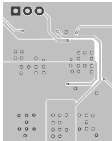
Inner Layer 2
