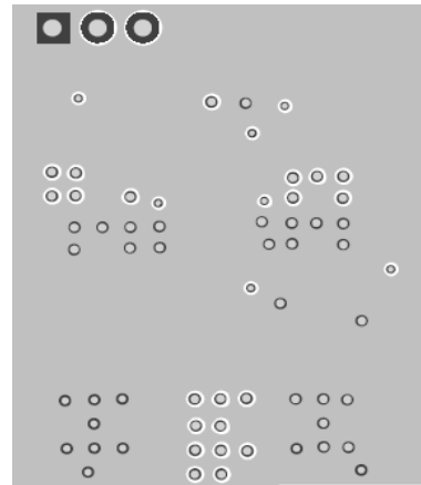
Inner Layer 1
