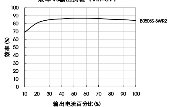
效率 Vs 输出负载 (Vin=5V)
