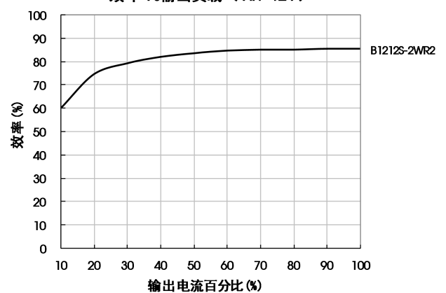
效率Vs输出负载 (Vin=12V)
