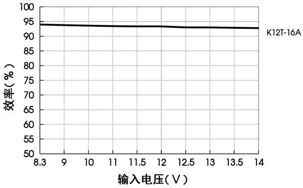
效率Vs输入电压 ( V_{out}=3.3V, I_o=16A )
