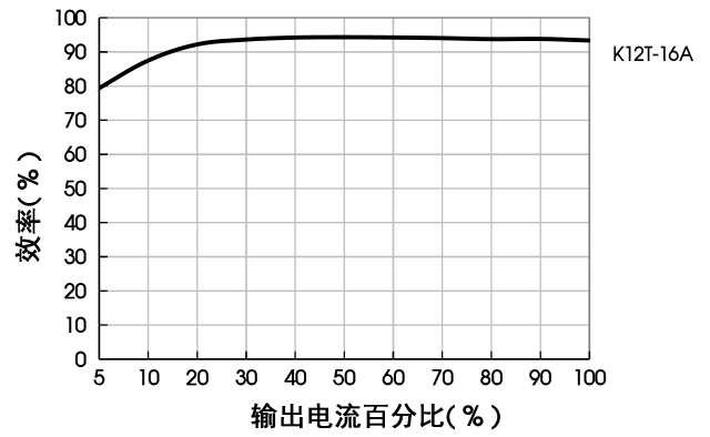
效率Vs输出负载 ( V_{in}=12V, V_{out}=3.3V )
