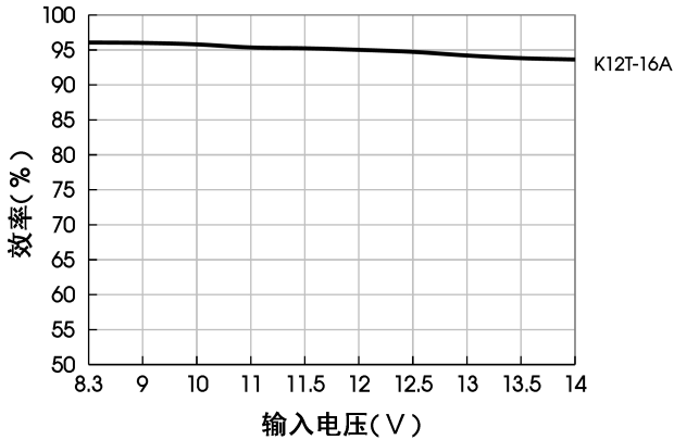
效率Vs输入电压 ( V_{out}=5V, I_o=16A )
