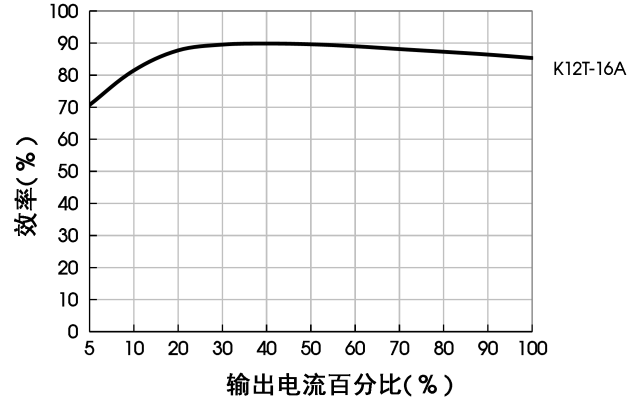
效率Vs输出负载 ( V_{in}=12V, V_{out}=1.2V )
