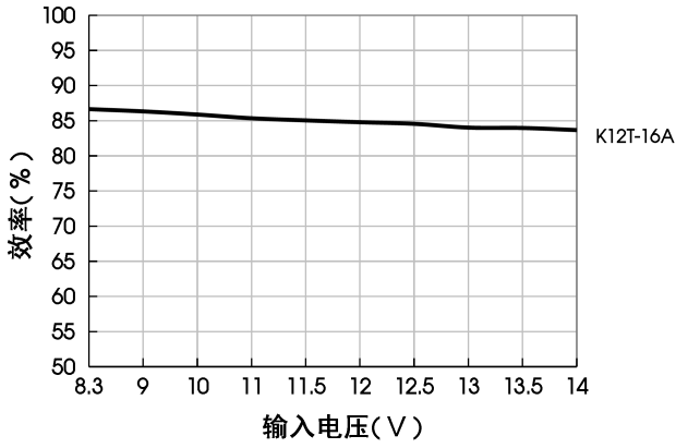
效率Vs输入电压 ( V_{out}=1.2V, I_o=16A )
