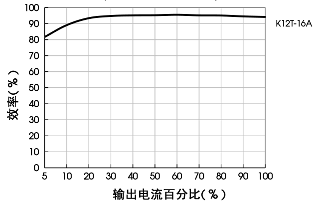
效率Vs输出负载 ( V_{in}=12V, V_{out}=5V )
