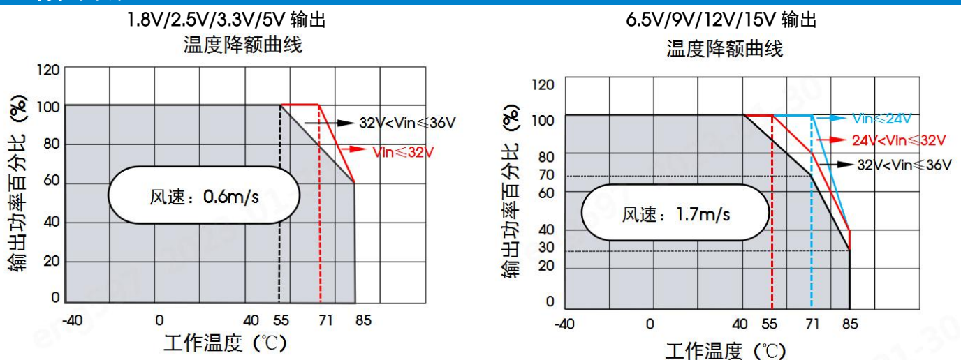
图 1-① 强制风冷曲线
