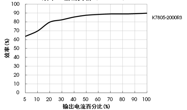
图 1-② 自然空冷曲线
