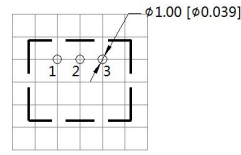
K78XX
