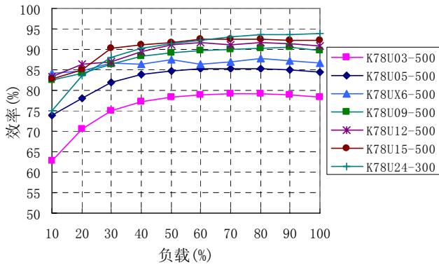
效率VS负载曲线图(Vin=Vin-nominal)
