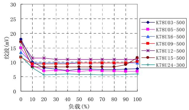
纹波VS负载曲线图(Vin=Vmin)
