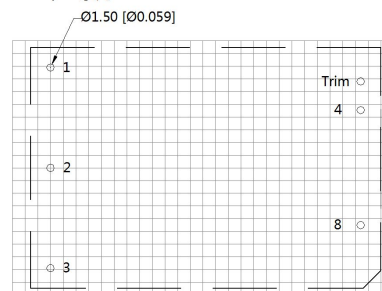
LH20/25系列
