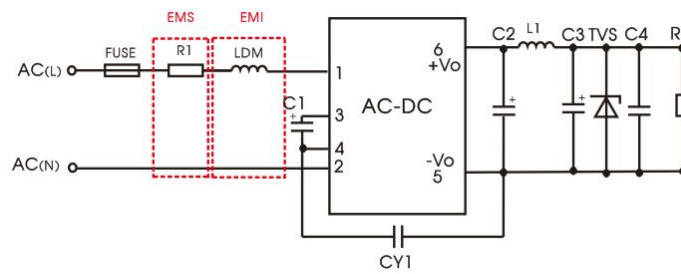
推荐电路 1
