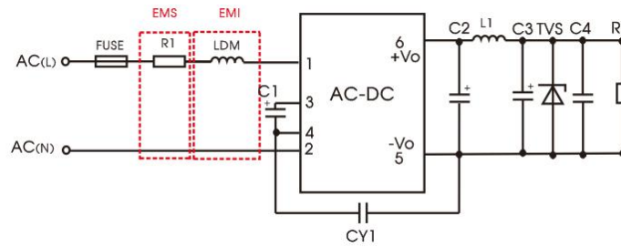
推荐电路 1
