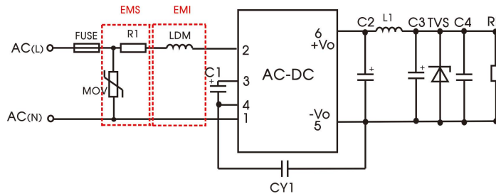
推荐电路 4
