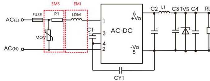
推荐电路 4
