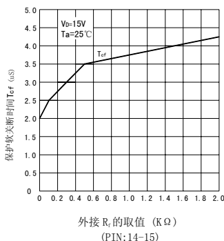
保护软关断时间与R f 关系的参考曲线
