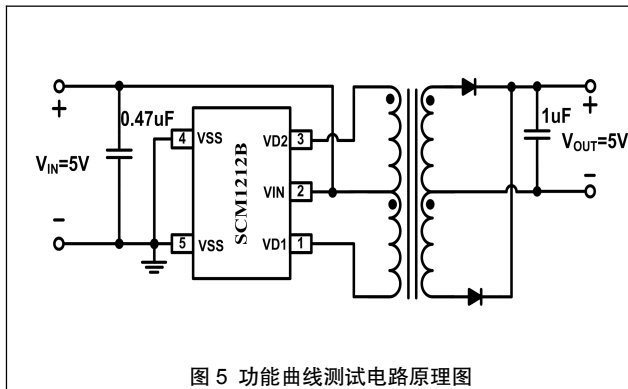
图5 功能曲线测试电路原理图
