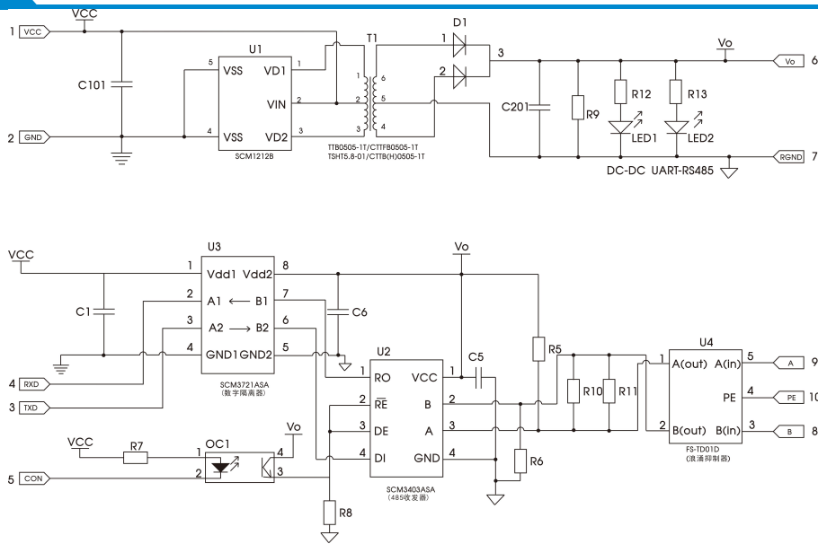
图 19 应用电路一
