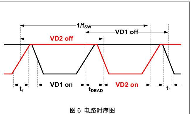
图6 电路时序图
