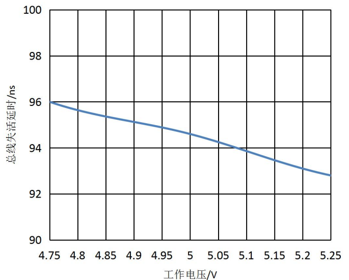
图4 总线失活延时 VS 工作电压
