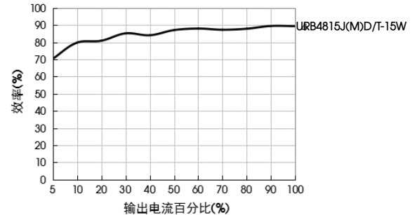
效率Vs输出负载 (Vin=48V)
