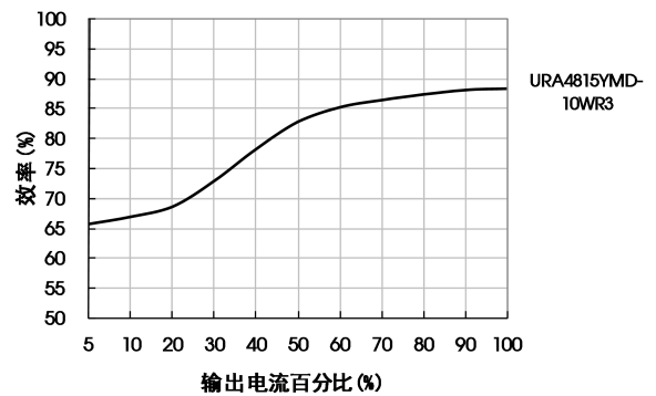
效率Vs输出负载 (Vin=48)
