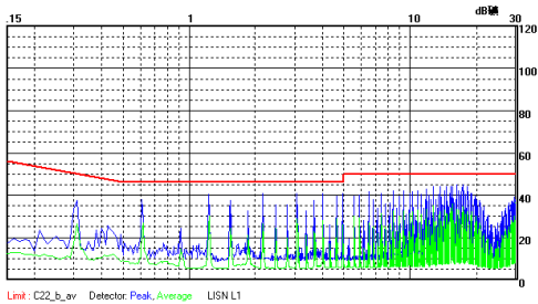
VRA2415YMD-6WR2 传导骚扰 Class B 测试效果图 (正线)
