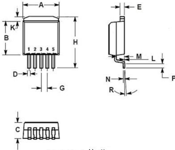
TO-263-5 外形
