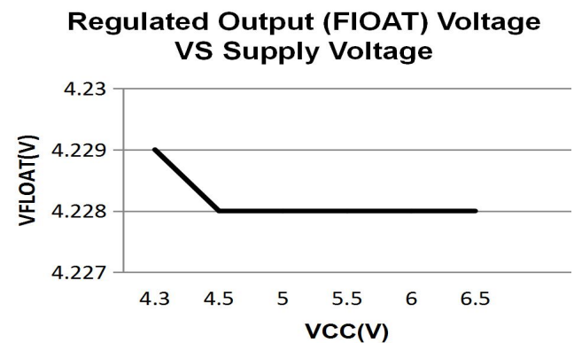
浮充电压与电源电压关系
