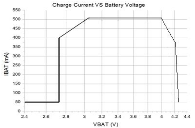
充电电压与充电电流关系
