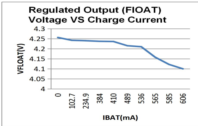
浮充电压与充电电流关系
