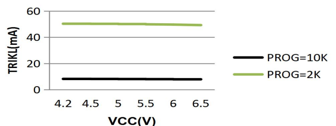
涓流电流与电源电压关系
