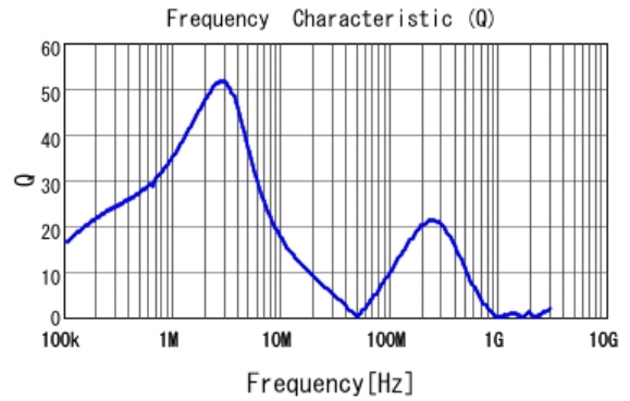
■ 1248AS-H-3R3N Q
