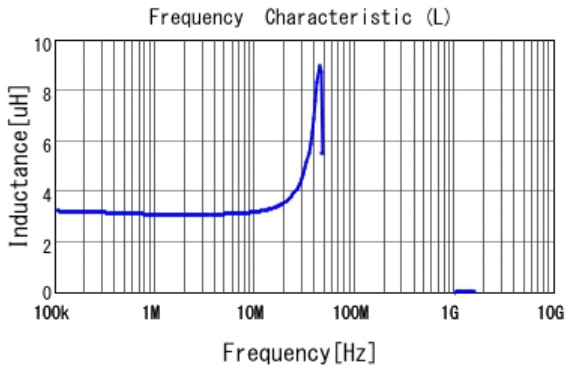
■ 1248AS-H-3R3N L
