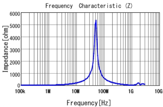
■ 1248AS-H-3R3N |Z|
