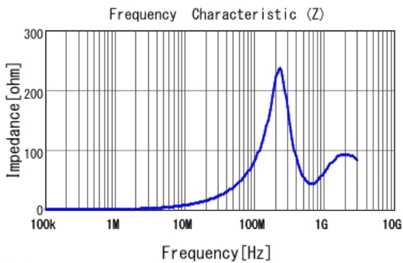
■ FDUE0630-H-R12M |Z|
